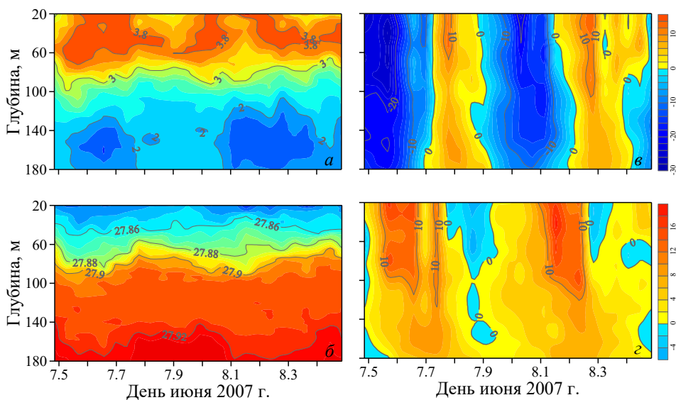
Рис. 6. Результаты измерений на суточной станции: температуры ( ^{\circ}\text{C} ) – a ; условной плотности ( \text{кг/м}^3 ) – b ; восточной компоненты скорости течения ( \text{см/с} ) – в ; северной компоненты скорости течения ( \text{см/с} ) – г
