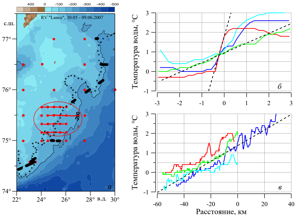
Рис. 4. Характеристики фронтального раздела по данным судовой метеостанции: a – гидрологические станции (красные точки), положение температурной фронтальной зоны (черные отрезки), зона размывтия фронтального раздела атлантических и арктических вод (красные линии, выделенные эллипсом), положение фронтальной зоны, восстановленное по рис. 3 (черные крестики); б – температура воды при пересечении фронтальной зоны; в – изменчивость температуры в зоне плавного раздела арктических и атлантических вод
