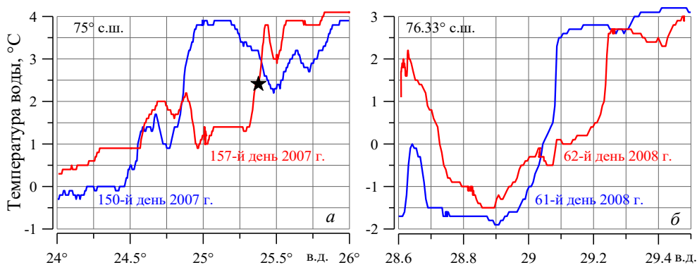
Рис. 5. Временная изменчивость положения фронтальной зоны на широтных разрезах в 2007 г. ( a ) и 2008 г. ( б ). Звездочка – место проведения суточной станции
