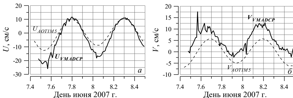
Рис. 8. Приливные течения: a – восточная компонента скорости течения (сплошная линия) и рассчитанная по модели AOTIM5 приливная составляющая M_2, S_2 (штриховая); б – то же самое для северной компоненты скорости течения
