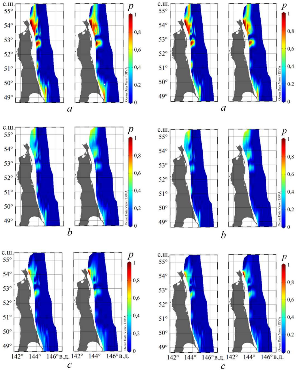
Рис. 5. Карты уровней вероятности превышения ( p ) для придонной (слева) и приповерхностной (справа) скоростей 0,25 м/с по абсолютному значению ( a ), в направлении к берегу ( b ) и от берега ( c ) Fig. 5. Maps of probability levels of exceeding ( p ) for the near-bottom (left) and near-surface (right) velocities 0.25 m/s according to the absolute values ( a ), towards the coast ( b ) and away from the coast ( c )
