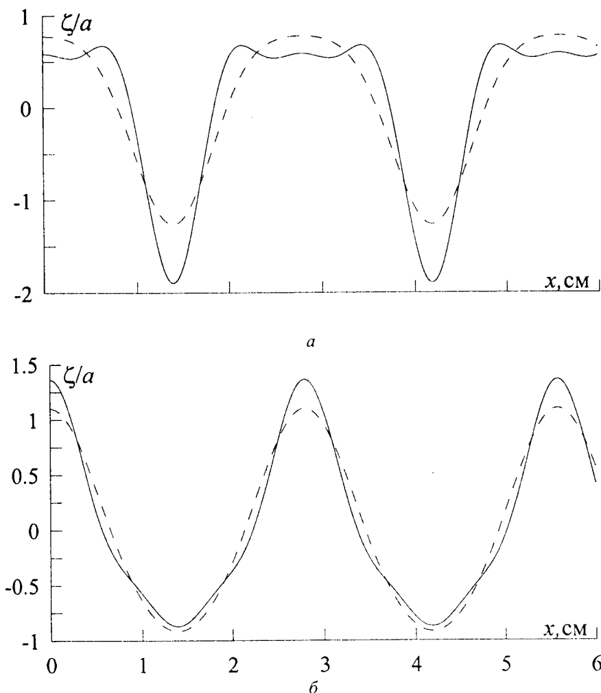
Р и с. 2. Профили волновых возмущений с учетом (штриховые линии) и без учета (сплошные) слагаемых F_2^0 , F_3^0 , L_3^0 для случая h = 0,55 см, k = 2,25 см -1 , a = 0,05 см, t = 0 при \alpha = 74 дин/см (а) и \alpha = 30 дин/см (б)
